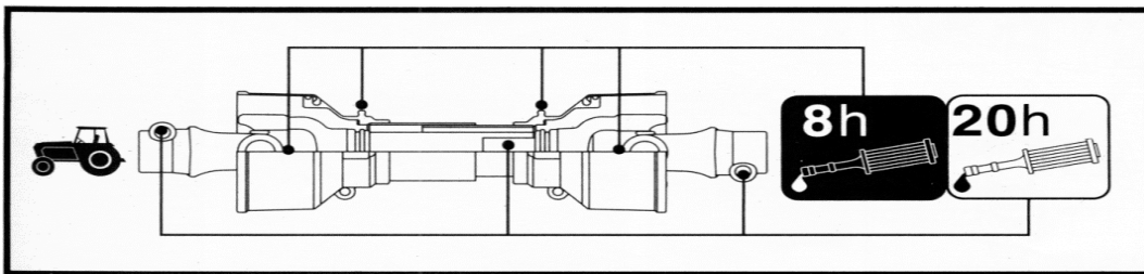
Rys. 15 Smarowanie wałka WPT
