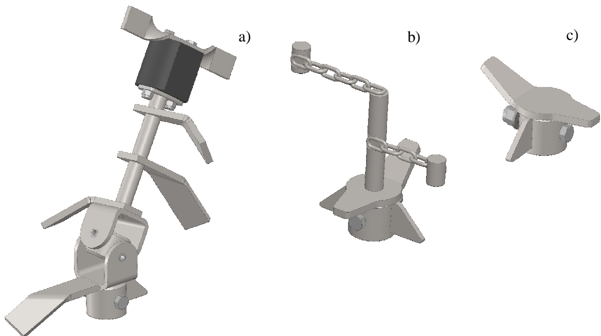
Rys. 3 Rodzaje mieszadeł, przeznaczenie: (a) piasek lub piasek z solą, (b) sól lub grys z solą, (c) grys, nawozy granulowane.
