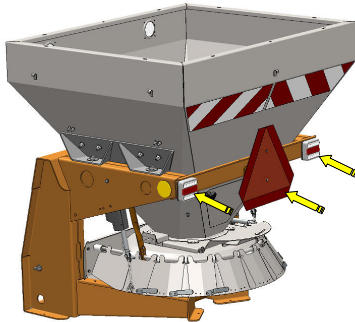
Rys.1 Rozmieszczenie urządzeń świetlnych.
